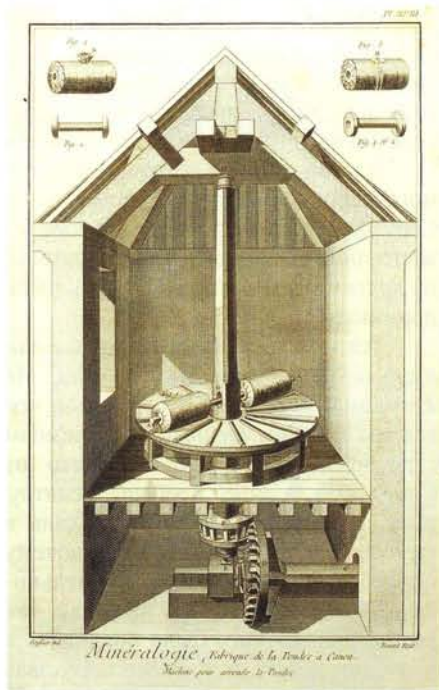
Схема мельницы для производства пушечного пороха
