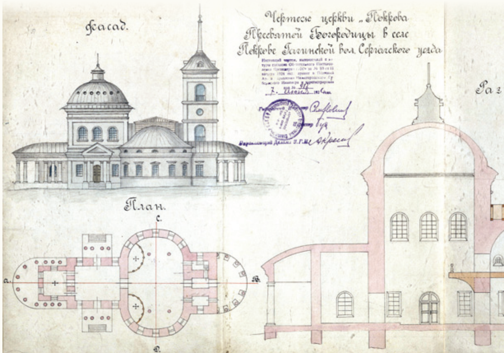
Чертёж Покровской церкви. 1925. Центральный архив Нижегородской области
