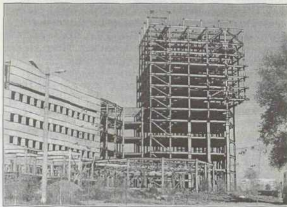
Каркас здания Центра микроэлектроники
